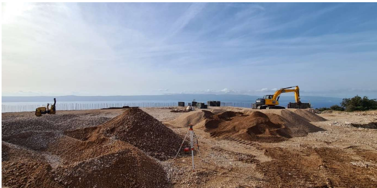
Slika 4: Prikaz radova na izgradnji Pretovarne stanice Brač (prosinac 2023.)
