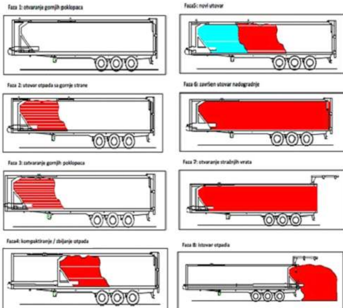
Slika 7. Prikaz faza rada: punjenje poluprikolice otpadom, zbijanje otpada, istovar otpada.
