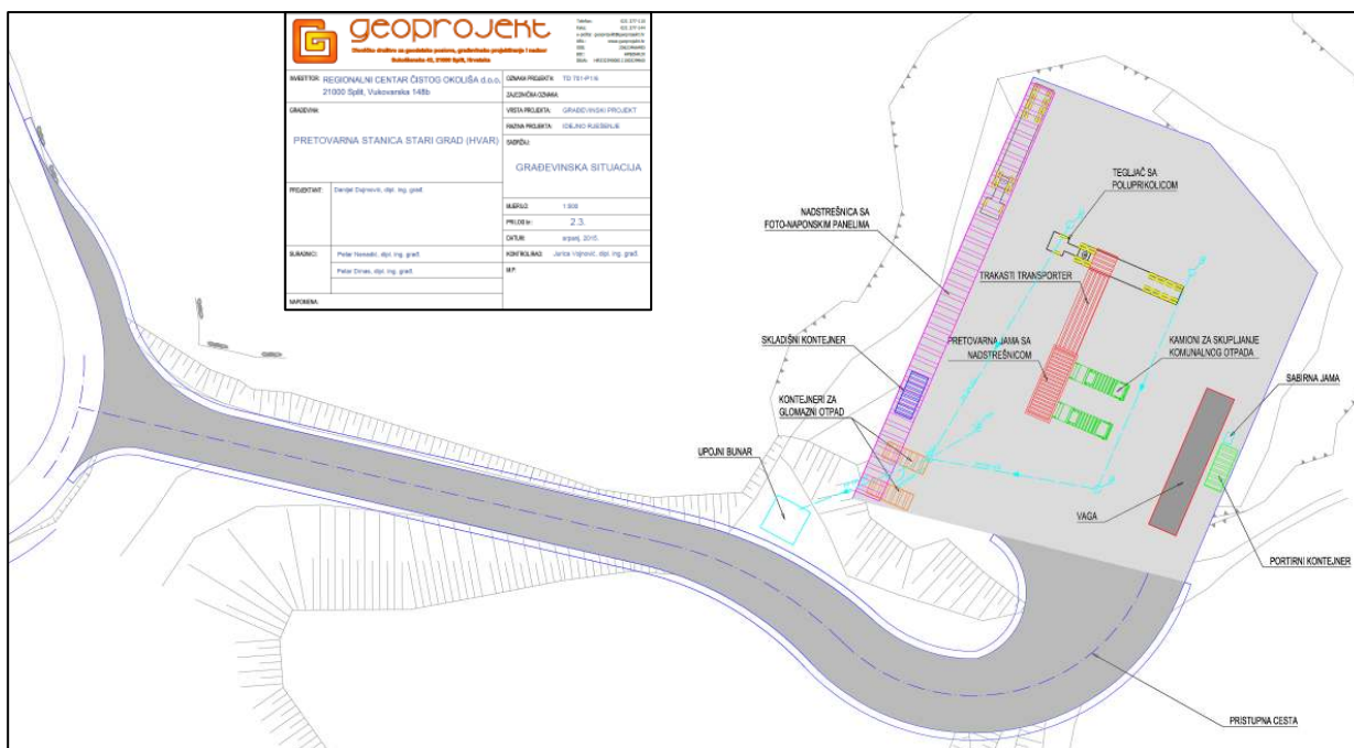
Slika 1. Idejno rješenje Pretovarne stanice Stari Grad na Hvaru. Geoprojekt d.d., Split, srpanj 2015.
