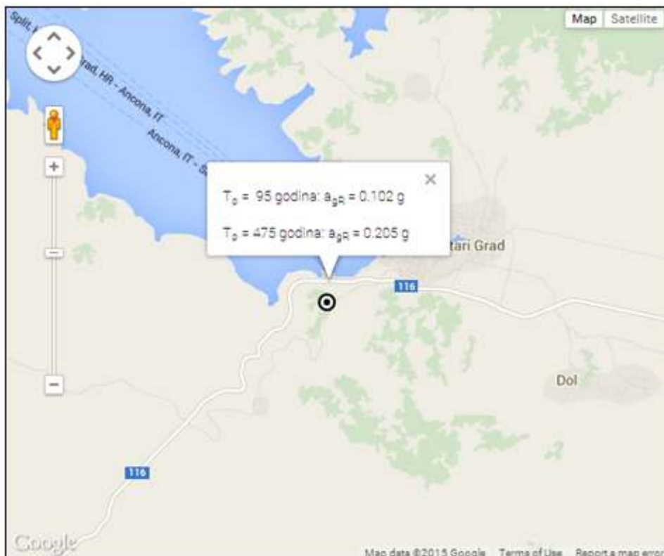
Slika 16. Iznos horizontalnih vršnih ubrzanja tla tipa A ( a_{gR} ) za povratna razdoblja od T_p=95 i 475 godina, izraženih u jedinicama gravitacijskog ubrzanja ( 1\text{ g} = 9.81\text{ m/s}^2 ), za područje zahvata. Izvor: seizkarta.gfz.hr (travanj 2015.)
