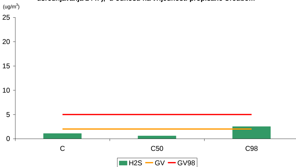
Statistički pokazatelji mjerenih vrijednosti koncentracije H_2S ( vrijeme usrednjavanja 24 h ), u odnosu na vrijednosti propisane Uredbom
