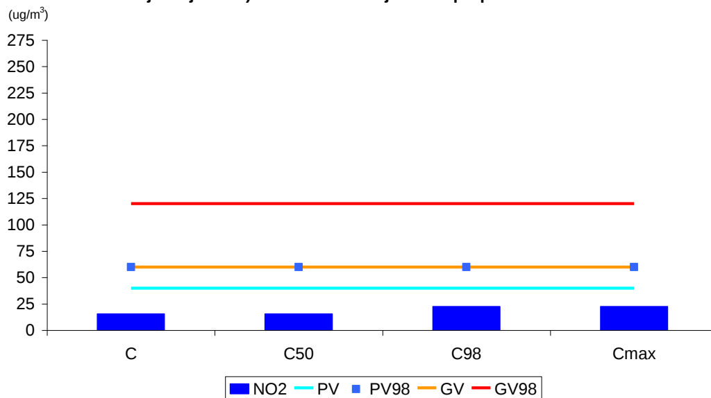
Statistički pokazatelji mjerenih vrijednosti koncentracije \text{NO}_2 ( vrijeme usrednjavanja 24 h ) u odnosu na vrijednosti propisane Uredbom
