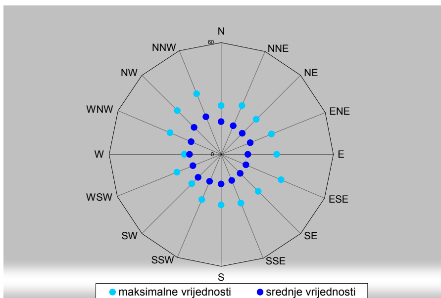
Slika–A.3.12.1/10 – Srednje i maksimalne vrijednosti \text{NO}_2 – vrijeme usrednjavanja 24 h
